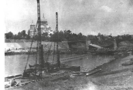
Воины Красной Армии ведут строительство нового обходного моста под нагрузку 60 тонн через реку Нерис. Вильнюс. Июль 1944
