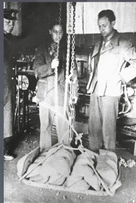
Испытание ножей для минных тралов на перерезание троса СССР, Ленинград, Балтийский судостроительный завод, 1943 Музей Победы
